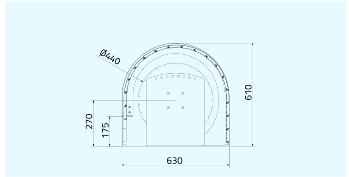
Verkleidungen ACOE Rollläden Größe 1
