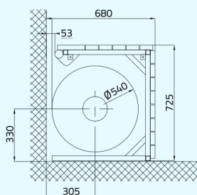
Größe 4 Wickeldurchmesser max. 600 mm
