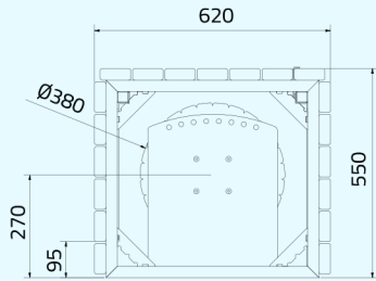
Größe 2 (2A, 2B, 2C, 2D, 2E) ACOE
