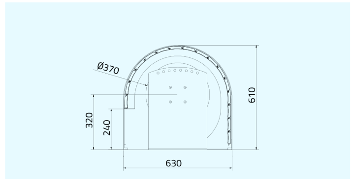
Verkleidungen ACOE Isola
