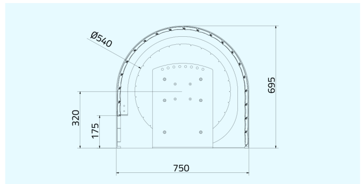
Verkleidungen ACOE Rollläden Größe 2
