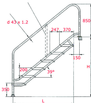
Bsp.: Treppe sechsstufig - 37.400.118
