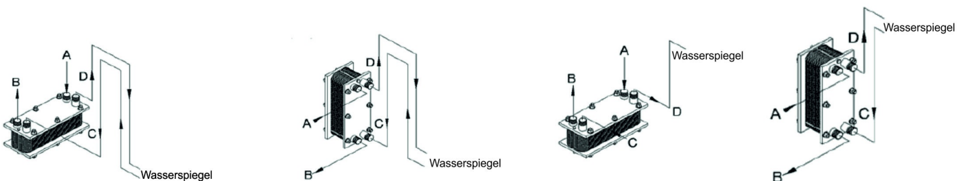
Installation oberhalb des Wasserspiegel
