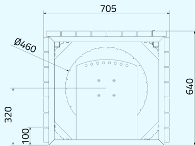
Größe 3 (3A, 3B, 3C, 3D, 3E) ACOE
