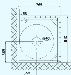
Größe 4 Wickeldurchmesser max. 600 mm
