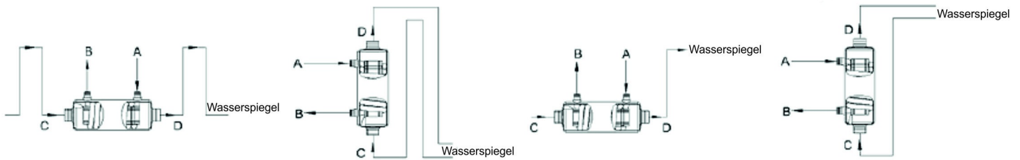
Installation oberhalb des Wasserspiegel
