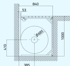
Größe 5 Wickeldurchmesser max. 685 mm
