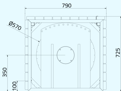
Größe 4 (4A, 4B, 4C, 4D, 4E) ACOE
